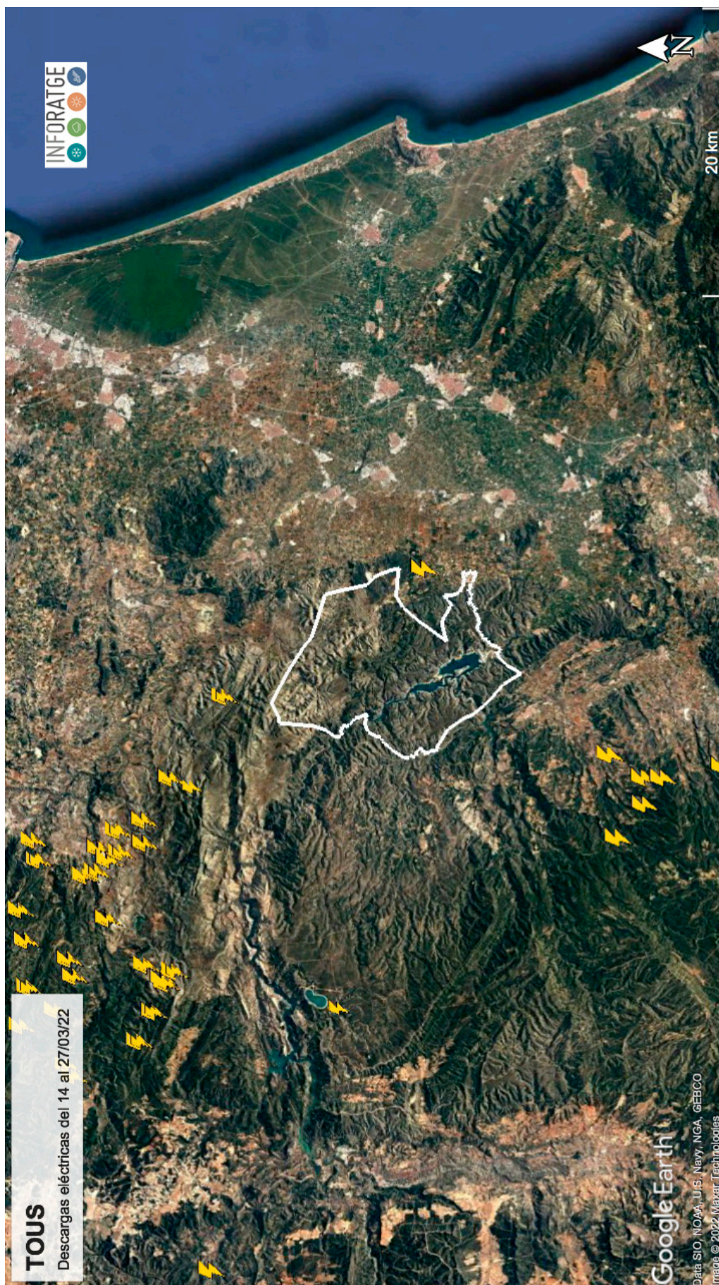
Geolocalización de las descargas eléctricas ` nube-tierra` registradas en el término municipal de TOUS entre el 14 y el 27/03/22 Fuente descargas eléctricas: AEMET, Agencia Estatal de Meteorología // Cartografía: © Instituto Geográfico Nacional de España
